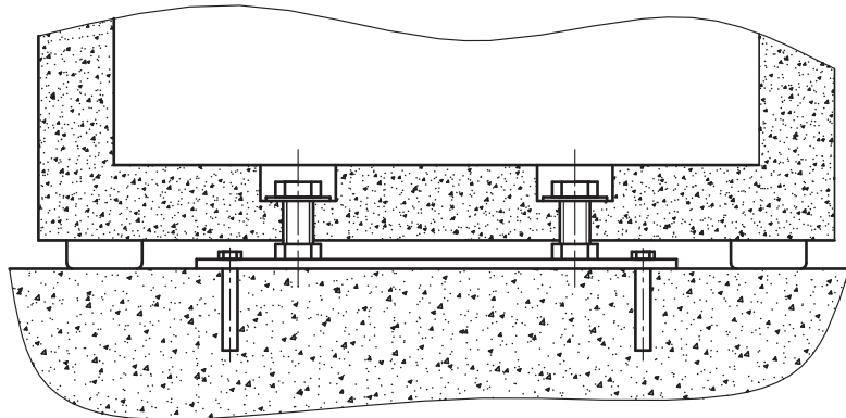
Схема крепления сейфа к полу
